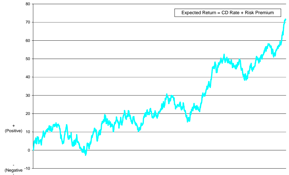
Drift & Diffusion
